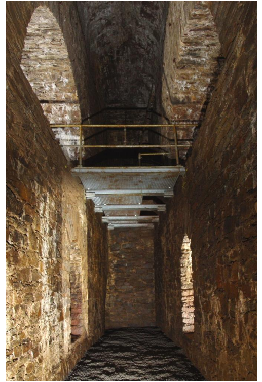
Radkammer am Kunstschaft Neu Gottes Geschick (Foto Vereinsarchiv)
